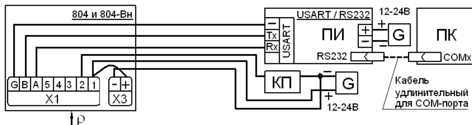
Рисунок В.7 - Схема подсоединения внешних электрических цепей плотномеров 804 и 804-Вн с выходными сигналами: цифровым USART и постоянного тока 4-20мА (см. рис.В.2; П ИИ – USART/RS232)
