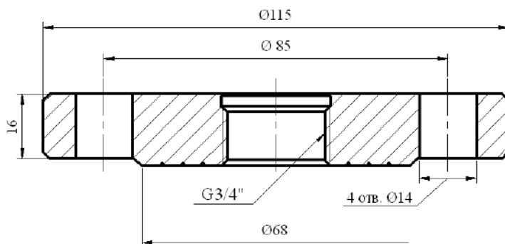
Рисунок А.7 - Фланец переходной Ду25 / G3/4 , P_y \leq 4 МПа
