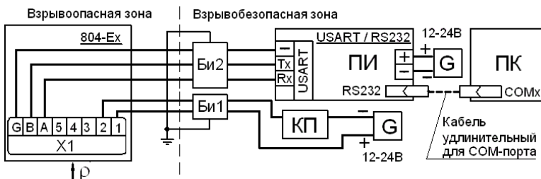
Рисунок В.14 - Схема подключения внешних электрических цепей плотномеров 804-Ex с выходными сигналами: цифровым USART и постоянным током 4-20мА (см. рис.В.2 и В.9; ПИ – USART/RS232)
