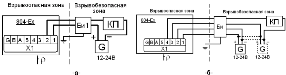
Рисунок В.13 - Схема подключения внешних электрических цепей плотномеров 804-Ex с выходным сигналом постоянного тока 4-20мА, варианты
